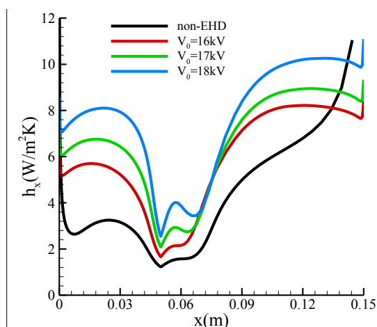
شکل ۱۶- توزیع ضریب انتقال حرارت موضعی روی پله پسرو با ولتاژهای مختلف ( a=6\text{cm} , Re=2122 )
