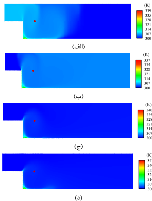
شکل ۱۴- توزیع دما در حضور میدان الکتریکی در اعداد رینولدز مختلف (a=۶cm) الف) Re=۳۴۲ (ب) Re=۷۵۳ (ج) Re=۲۱۲۲ (د) Re=۲۹۴۳
