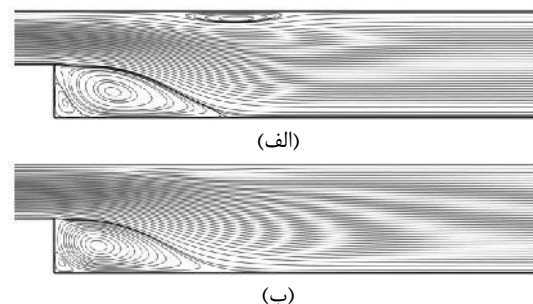
شکل ۱۰- خطوط جریان بدون حضور میدان الکتریکی ( a=6\text{cm} ) (الف) Re=753 (ب) Re=2122
