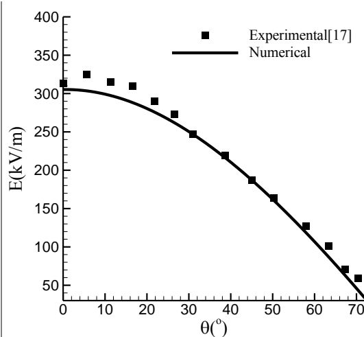
شکل ۶- مقایسه توزیع میدان الکتریکی حاصل از تحلیل عددی و نتایج تجربی ( V_0=18\text{kV} )
