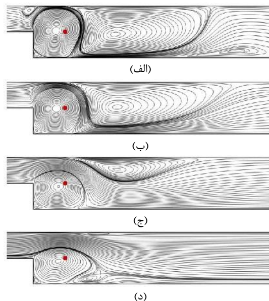
شکل ۱۳- خطوط جریان در حضور میدان الکتریکی (a=۶cm, V_0=18kV )
