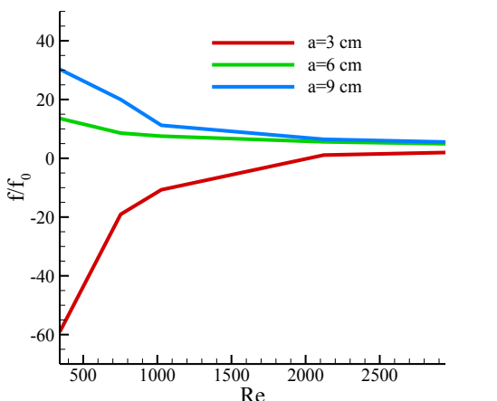
شکل ۲۲- نسبت ضریب اصطکاک در فواصل مختلف الکتروود از پله در V_0=18kV
