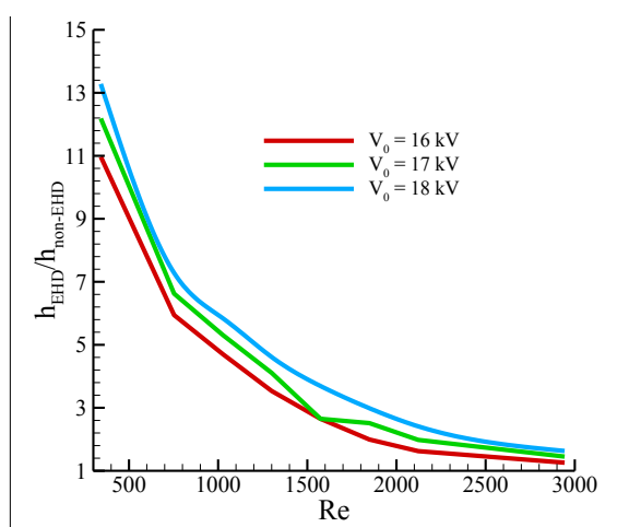
شکل ۱۷- نسبت افزایش ضریب انتقال حرارت در اعداد رینولدز و ولتاژهای اعمالی مختلف ( a=6\text{ cm} )
