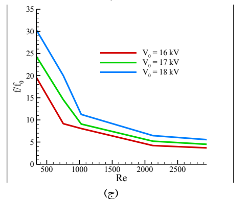
شکل ۲۱- نسبت ضریب اصطکاک در اعداد رینولدز و ولتاژهای اعمالی مختلف
