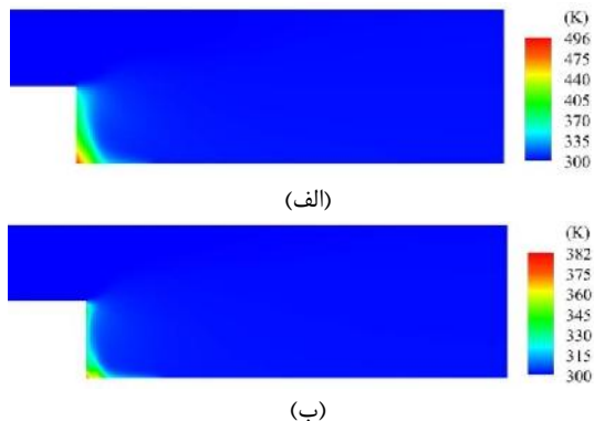
شکل ۱۱- توزیع تابع دما در حالت عدم حضور میدان الکتریکی ( a=6\text{cm} ) (الف) Re=753 (ب) Re=2122
