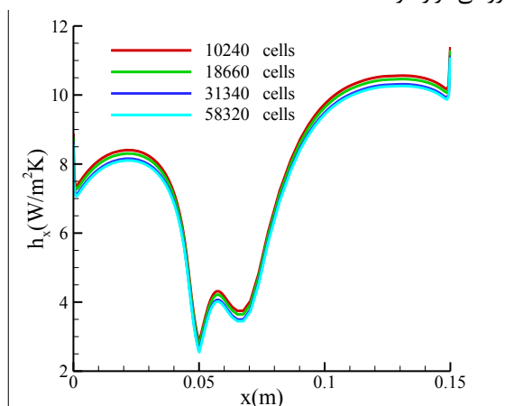
شکل ۳ - بررسی استقلال از شبکه، (a=۶cm)
