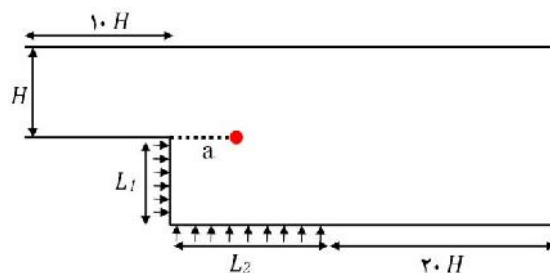
شکل ۱- هندسه و دامنه محاسباتی مدل
