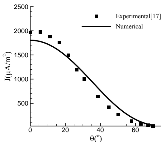
شکل ۷- مقایسه توزیع چگالی جریان الکتریکی حاصل از تحلیل عددی و نتایج تجربی ( V_0=18\text{kV} )
