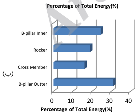
شکل ۲۳- درصد جذب انرژی قطعات بدنه منفصل خودرو در برخورد از جانب در مدل شرکت پورشه [۱۵] (الف) و پلتفرم (ب)
