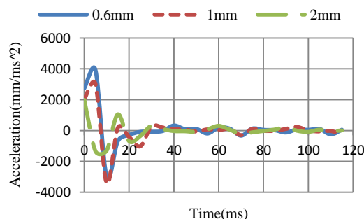
شکل ۳۰- نمودار شتاب قطعه ستون میانی در ضخامت‌های مختلف این قطعه در برخورد از جانب با سرعت ۱۵ متر بر ثانیه
