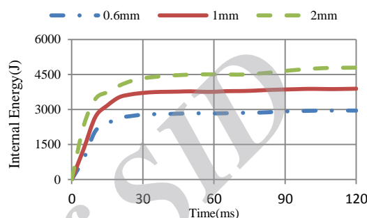
شکل ۲۹- نمودار تغییرات انرژی درونی قطعه ستون میانی در ضخامت‌های مختلف این قطعه در برخورد از جانب با سرعت ۱۵ متر بر ثانیه
