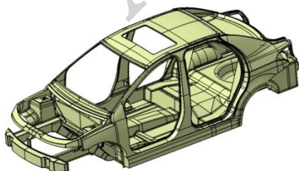
شکل ۱۲- مدل کامل بدنه منفصل خودرو کلاس B
