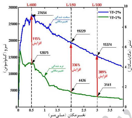
شکل ۷- منحنی مقایسه ای نیرو- تغییر مکان و تنش- تغییر مکان نمونه های مسلح به ۱ و ۲ درصد ییاف
