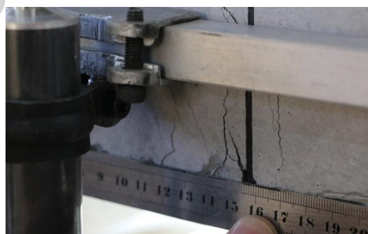
شکل ۱۳- ترک خوردگی‌های متعدد نمونه‌ها
