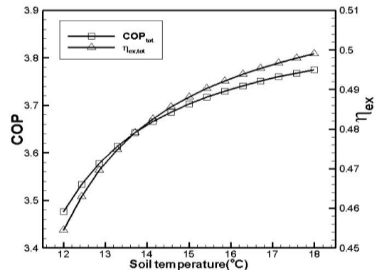
شکل ۹- اثر تغییر دمای خاک بر ضریب عملکرد و بازده انرژی
