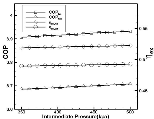
شکل ۶- اثر تغییر فشار میانی سیکل بر ضریب عملکرد و بازده انرژی
