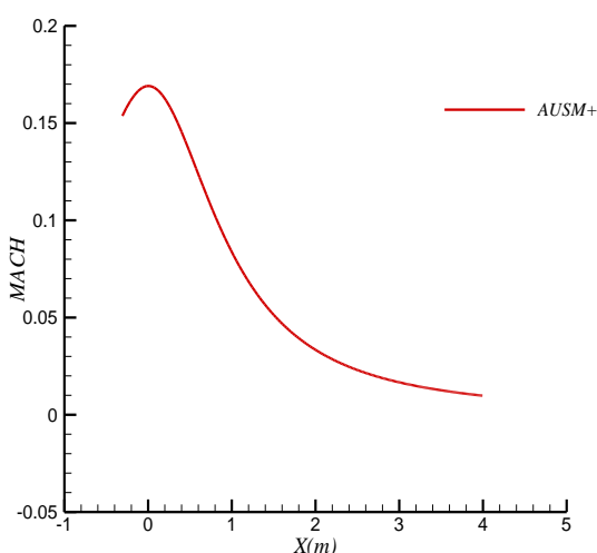
شکل ۸- نمودار عدد ماخ در داخل نازل (نسبت فشار = ۰/۹۹۶)
