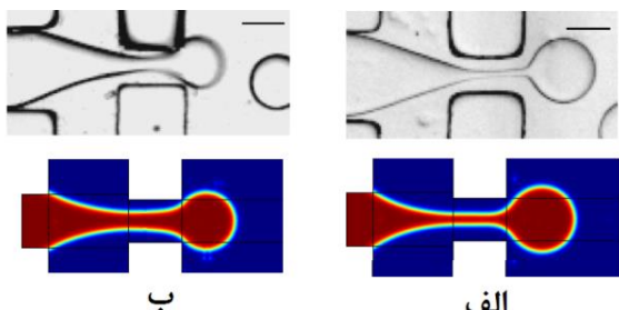
شکل ۱۰- تصاویری از شکل‌گیری قطره بر اساس نتایج تجربی (بالا) [۵۶] و نتایج شبیه‌سازی (پایین) در شرایط Q_c/Q_d = 20 و Q_d = 0.04 \text{ mL/h} برای دو مقدار مختلف از ویسکوزیته روغن معادل الف) 100 \text{ mPa.s} ب) 20 \text{ mPa.s}
