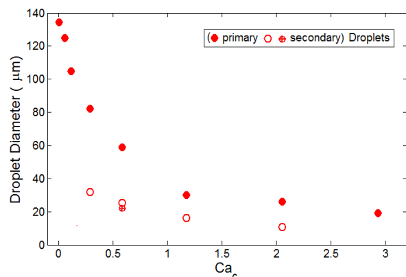
شکل ۱۵- قطر ریزقطرات روغن سیلیکون بر حسب عدد موئینگی فاز پیوسته
