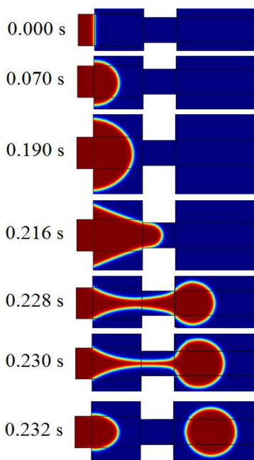
شکل ۶- فرآیند شکل‌گیری قطره برای نسبت Q_c/Q_d = 10 در دبی ثابت ۰/۰۴ \text{ mL/h} برای فاز گسسته
