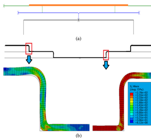
شکل ۷- پرشدگی گوشه قالب در قالب دوپله‌ای جدید
