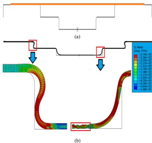
شکل ۶- پرشدگی گوشه قالب در قالب سنتی
