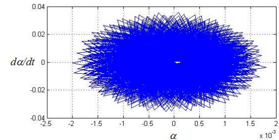
شکل ۶- نتایج شبیه سازی و نمودار فازی برای نسبت سرعت (۰/۷) در جریان پایا
