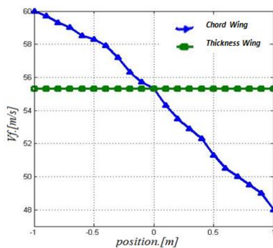
شکل ۵- موقعیت مخزن در جریان پایا
