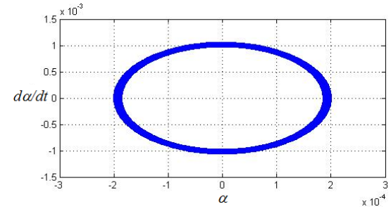
شکل ۷- نتایج شبیه سازی و نمودار فازی برای نسبت سرعت (۱) در جریان پایا
