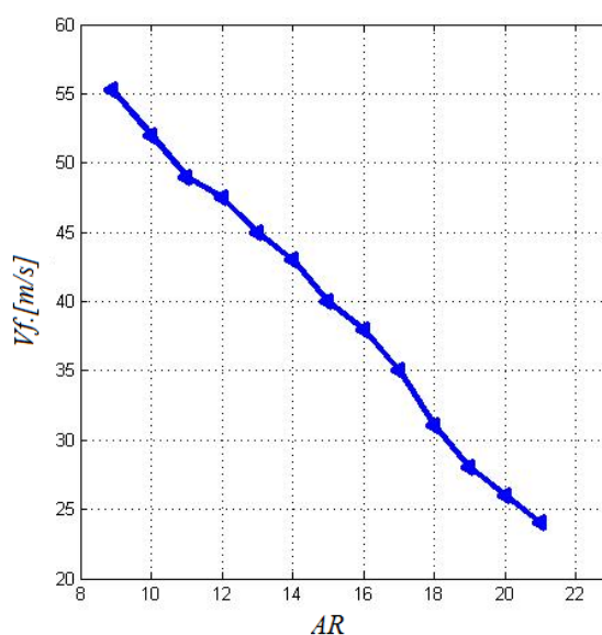
شکل ۴- تغییرات سرعت فلاتر بر حسب نسبت منطری
