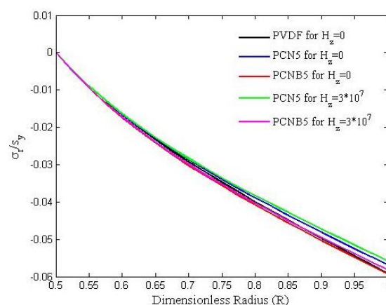
شکل ۱۸- نمودار تنش شعاعی در شرایط مرزی آزاد- ثابتو مقادیر مختلف اختلاف پتانسیل الکتریکی
