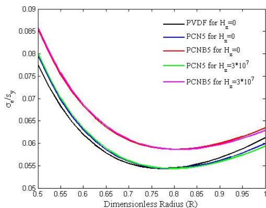
شکل ۱۶- نمودار تنش موثر در شرایط مرزی آزاد- ثابتمقادیر مختلف اختلاف پتانسیل الکتریکی
