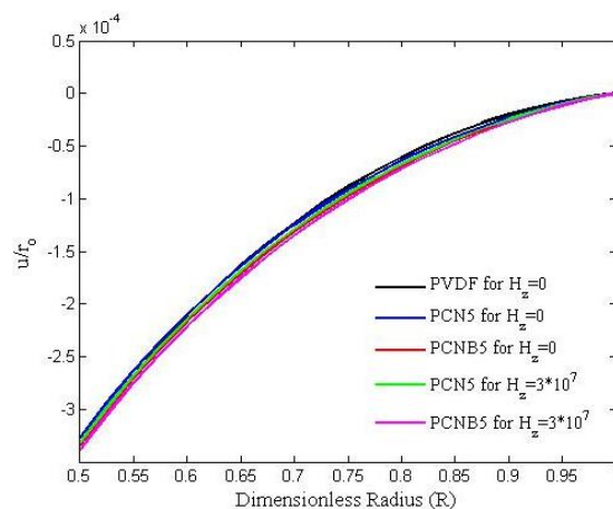
شکل ۱۷- نمودار جابجایی شعاعی در شرایط مرزی آزاد- ثابتو مقادیر مختلف اختلاف پتانسیل الکتریکی
