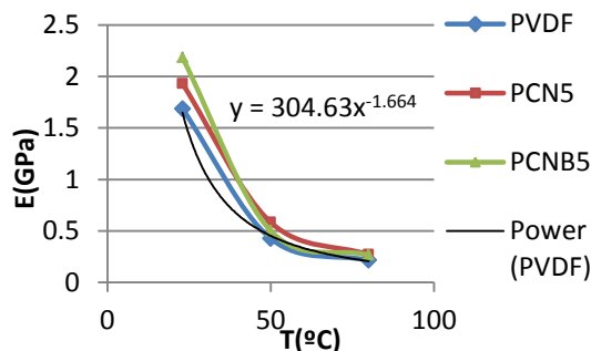
شکل ۵- نمودار تغییرات مدول الاستیسیته ماکسول با دما در تنش ۱۵ مگاپاسکال
