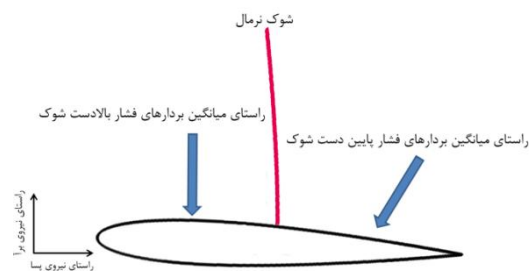
شکل ۱۵- اثرات هندسه بالادست و پایین‌دست شوک
