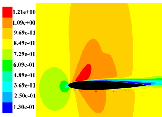
شکل ۱۱- کانتور عدد ماخ بعد از کنترل غیرفعال (میزان تخلخل ۵ درصد)
