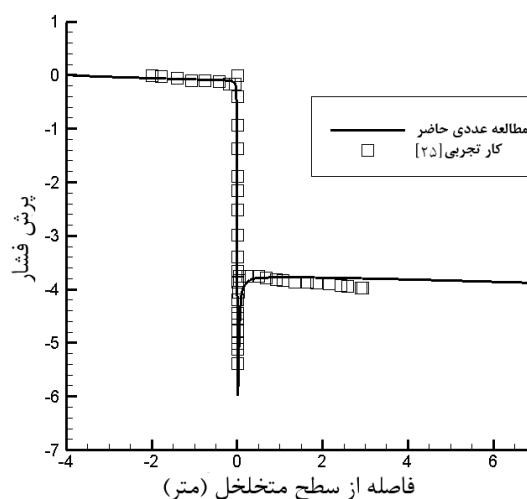
شکل ۹- مقایسه نتایج عددی و تجربی سطح متخلخل در مسیر جریان
