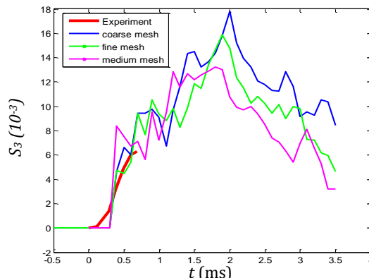
شکل ۸- مقایسه‌ی نمودارهای کرنش در محل حس گر S3 مدل اجزای محدود و آزمایش لیدو در حین برخورد
