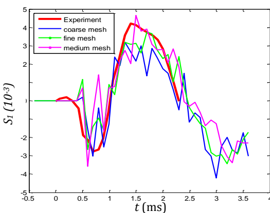
شکل ۶- مقایسه نمودارهای کرنش در محل حس گر S_1 مدل اجزای محدود و آزمایش لیو در حین برخورد
