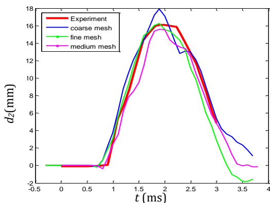
شکل ۵- مقایسه نمودارهای تغییر مکان در محل حس گر d_2 مدل اجزای محدود و آزمایش لیو در حین برخورد
