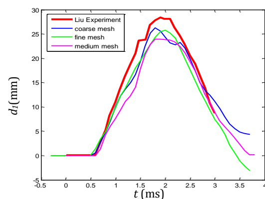
شکل ۴- مقایسه نمودارهای تغییر مکان در محل حس گر d_1 مدل اجزای محدود و آزمایش لیو در حین برخورد
