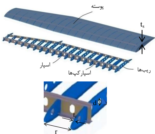
شکل ۹- اجزای سازه‌ی بال هواپیما
