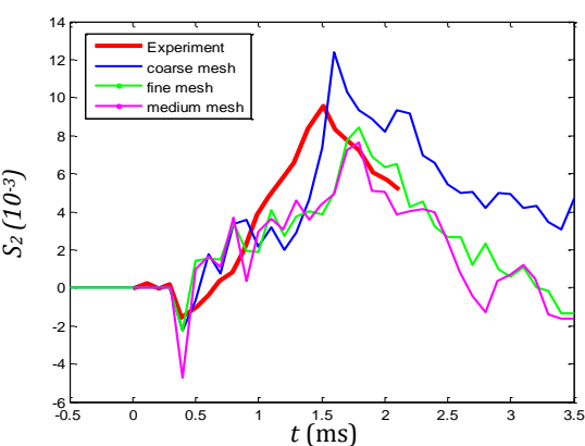
شکل ۷- مقایسه نمودارهای کرنش در محل حس گر S_2 مدل اجزای محدود و آزمایش لیو در حین برخورد
