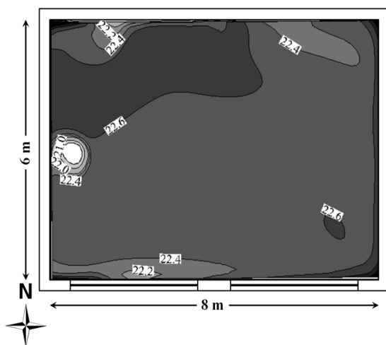
شکل ۱۰- توزیع دما (درجه سلسیوس) در ارتفاع ۱/۱ متری از کف به ازای قرارگیری دریاچه تأمین هوای تازه در موقعیت شماره ۳
