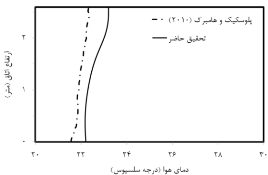
شکل ۵- صحت‌سنجی حل عددی با نتایج تحقیق پلوسکیک و هامبرگ [۱] برای توزیع دما در مرکز اتاق
