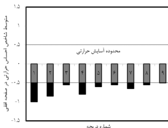
شکل ۸- متوسط شاخص آسایش حرارتی افراد در اتاق به ازای موقعیت‌های مختلف برای دریاچه تأمین هوای تازه
