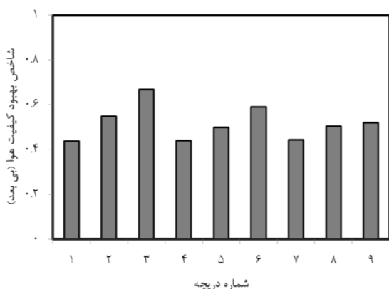
شکل ۹- متوسط شاخص بهبود کیفیت هوا در ناحیه تنفس به ازای موقعیت‌های مختلف برای دریاچه تأمین هوای تازه
