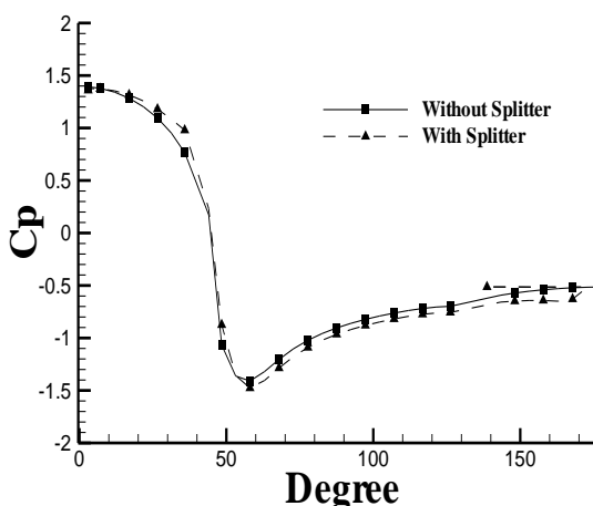
شکل ۱۶- مقایسه ضریب فشار حول استوانه بدون صفحه جداکننده و با صفحه جداکننده برای اختلاف ولتاژ 10kV
