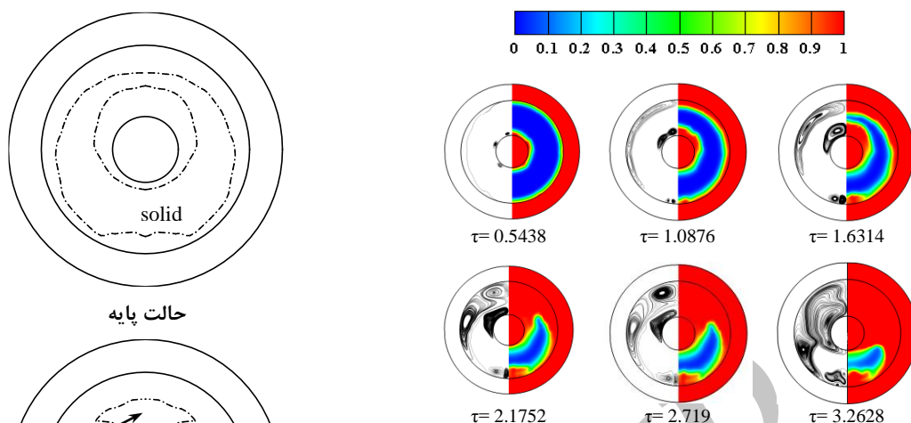
شکل ۸- کانتور کسر مایع و خطوط جریان در مقطع میانی مبدل حرارتی سه لوله‌ای
