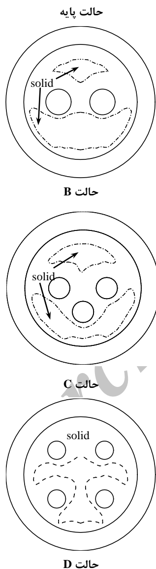
شکل ۹- موقعیت جبهه ذوب مبدل حرارتی سه لوله‌ای برای حالت‌های مختلف در \tau = 1.6314
