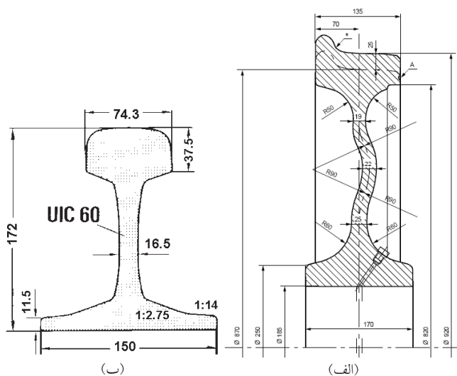
شکل ۲. (الف) نقشه سطح مقطع چرخ منبولوک با قطر ۹۲۰ میلی متر، (ب) نقشه سطح مقطع ریل UIC 60 [۱۱۰ و ۱۱].
