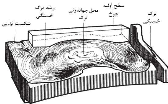
شکل ۱. چگونگی رشد ترک خستگی ایجاد شده در عمق ۴ میلی‌متری [۳]
