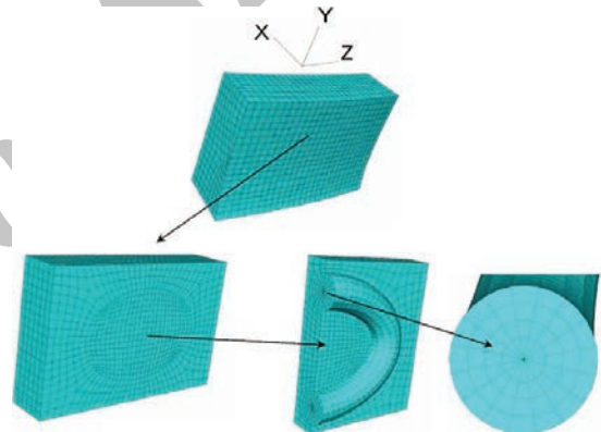
شکل ۶. چگونگی المان‌بندی قطاع حاوی ترک و جبهه ترک.
