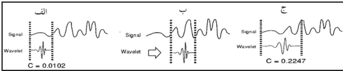
شکل ۲. مراحل انجام تبدیل موجک [Matlab 7.6.0]
