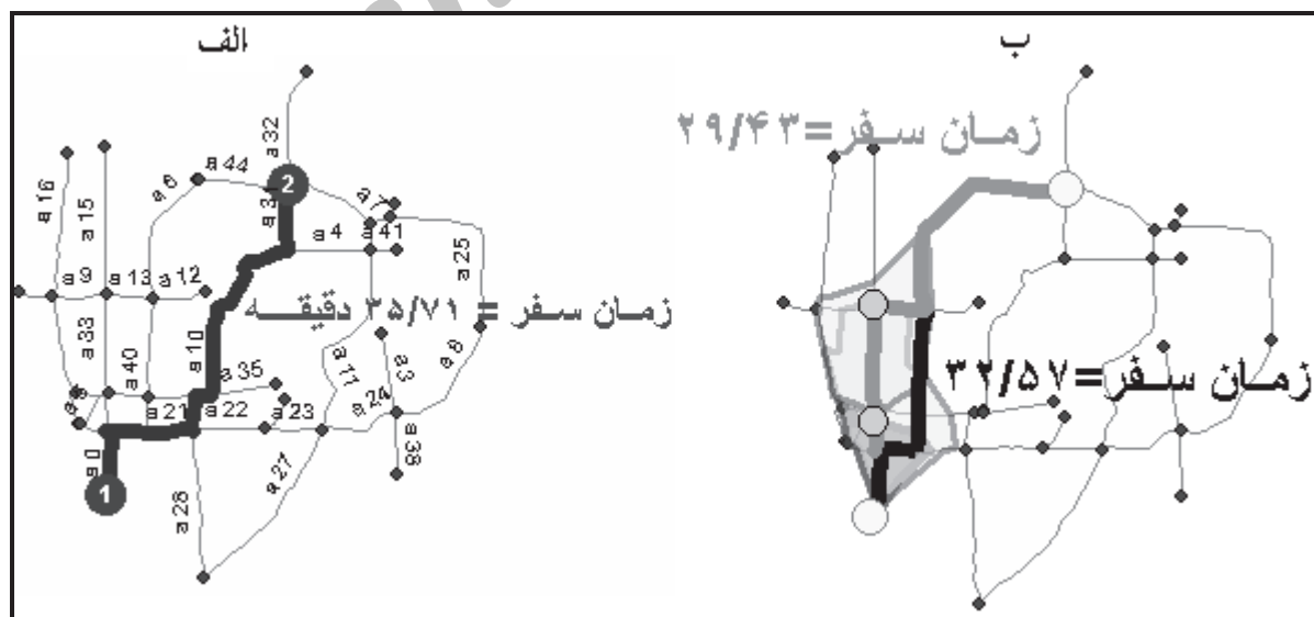
شکل ۷. نتایج مسیریابی دایجسترا بین گره ۸ و ۲۸ (الف) مسیریابی دایجسترا با در نظر گرفتن وزن ثابت برای یالها ب) مسیر به دست آمده از وزن آماری یالها (سیاه) و مسیر به دست آمده از وزن آماری و ریسک و تجزیه فضا زمان (خاکستری)
