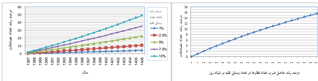
شکل ۳. روند درصد رشد تعداد تصادفات با درصد رشد حاصل ضرب تعداد قطارها در وسایل نقلیه در شبانه روز شکل ۴. درصد رشد تعداد تصادفات با درصد رشد سالانه تعداد وسایل نقلیه جاده‌ای بر اساس مدل ۲۲. (با فرض عدم تغییر دیگر متغیرها)
