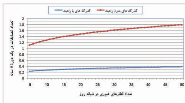
شکل ۱. روند تغییر تعداد تصادفات با تعداد وسایل نقلیه عبوری در شبانه‌روز بر اساس مدل ۲۲. (محاسبه شده با: تعداد وسایل نقلیه عبوری در شبانه‌روز = 1000 ، موقعیت گذرگاه برون‌شهری، متوسط سرعت قطارها بیش از 60 \text{ km/h} ، نوع روسازی جاده = آسفالتی)
