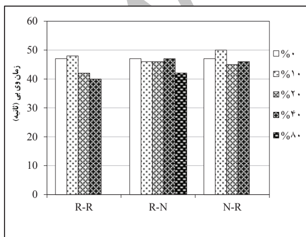
شکل ۱۲. زمان وی.بی در قبال درصدهای مختلف خرده آسفالت بازیافتی برای نسبت اختلاط شماره ۱
