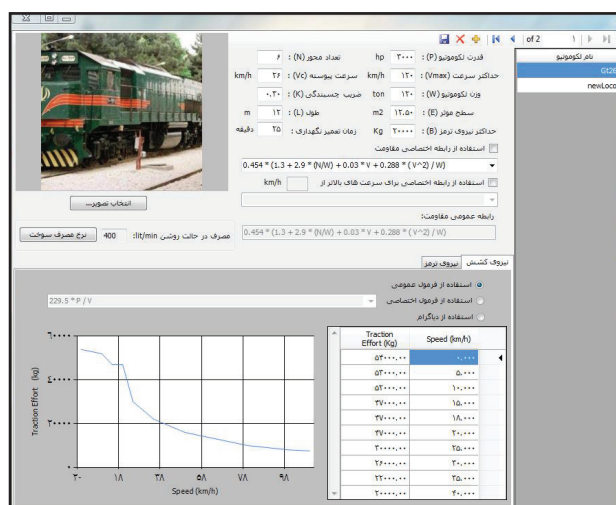
شکل ۸. صفحه مشخصات لکوموتیو GT26
