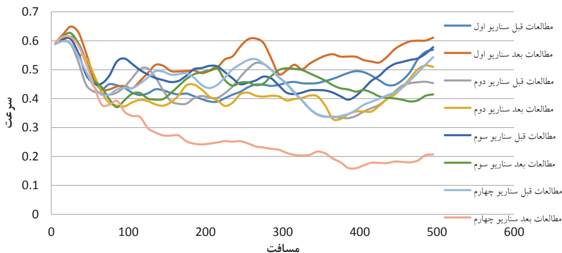
شکل ۵. نمودار پروفیل های جابجایی جانبی مطالعات قبل و بعد در هر دو سناریو
