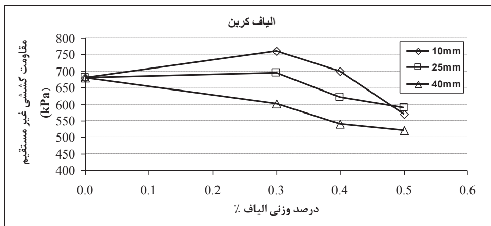
شکل ۹. تغییرات مقاومت کششی غیر مستقیم با مقدار الیاف کربن
