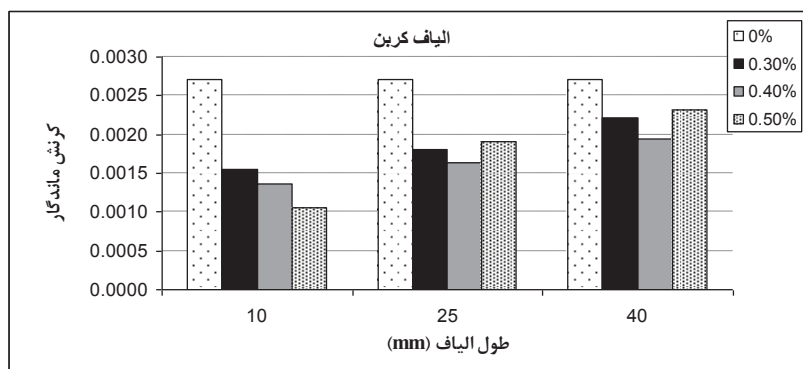
شکل ۱۶. تغییرات کرنش ماندگار با طول و مقدار الیاف کربن
