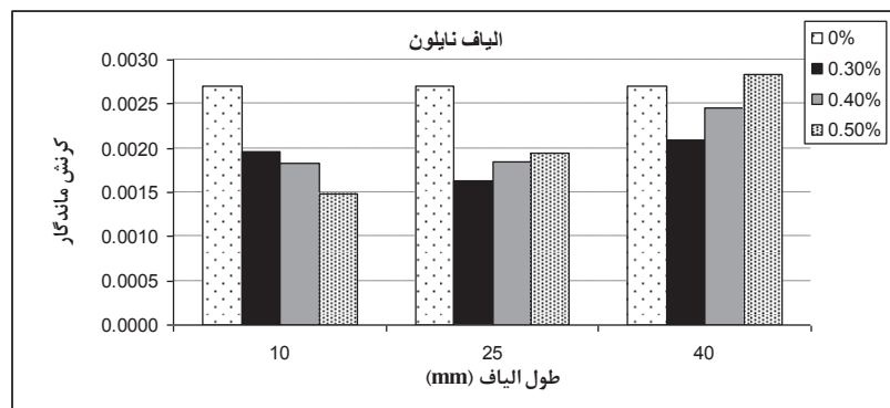
شکل ۱۷. تغییرات کرنش ماندگار با طول و مقدار الیاف نایلون
