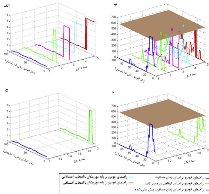
شکل ۱۰. کنترل ترافیک متمرکز بین شبکه و وسایل نقلیه: (الف) مجموع عبور و مرور لحظه‌ای (ب) مقایسه برنامه زمان‌بندی شبکه با ظرفیت مسیره‌ها. (ج) مجموع عبور و مرور لحظه‌ای و تراکم عبور و مرور در هر گام از تکرار و (د) مقایسه برنامه زمان‌بندی شبکه در هر گام با ظرفیت مسیره‌ها
