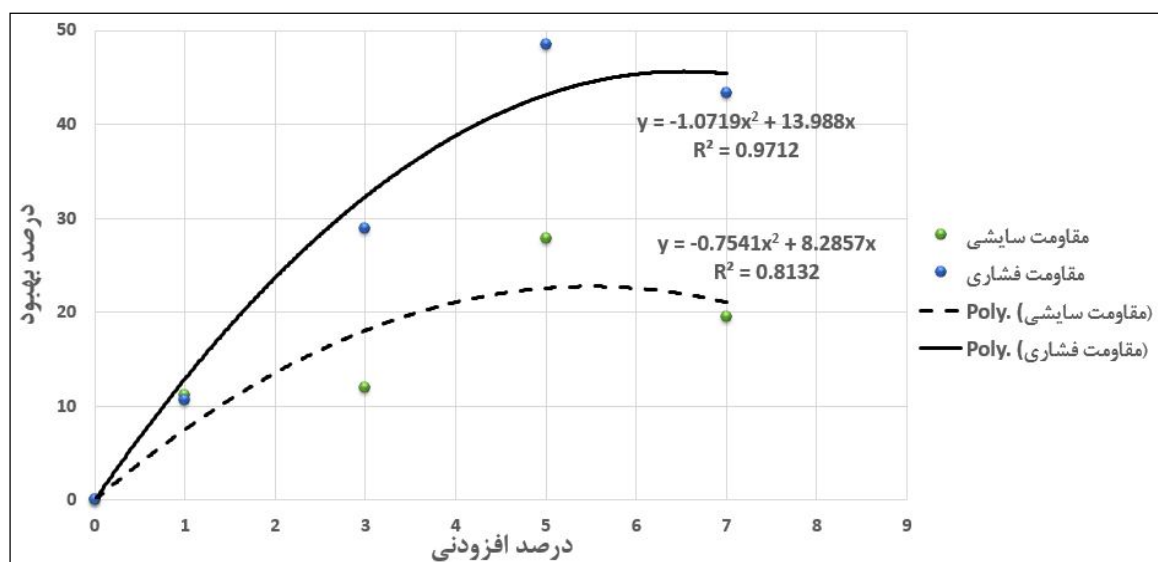
شکل ۴. مقایسه نتایج مقاومت فشاری و شاخص سایش برای پنج نوع مخلوط
