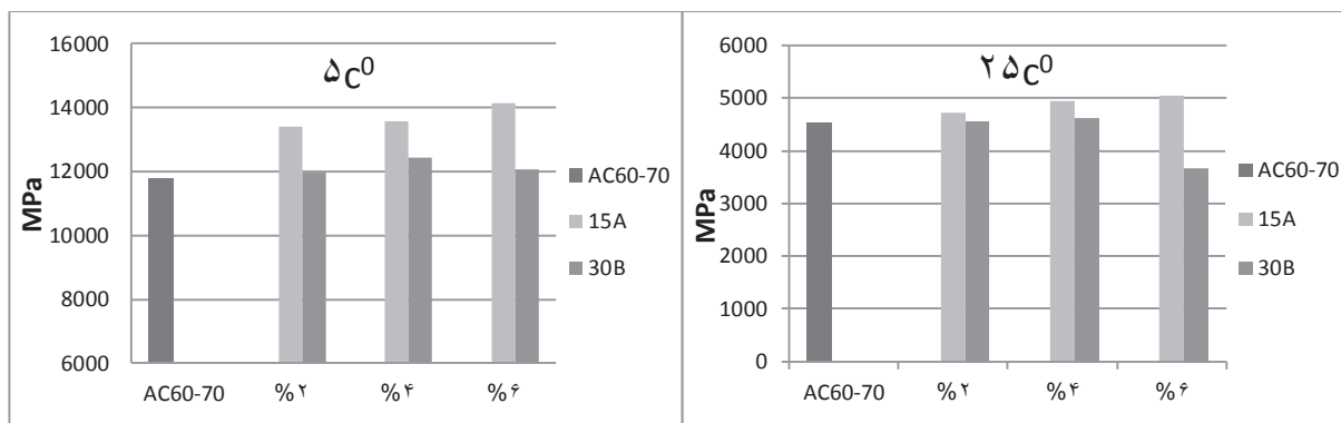
شکل ۶. نتایج آزمایش مدول برجهنگی در دمای ۲۵ و ۵ درجه سانتی‌گراد
