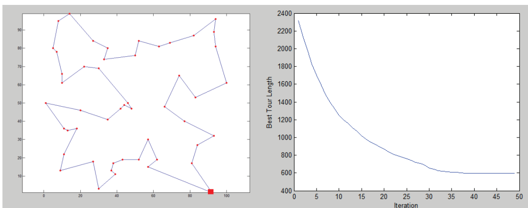
شکل ۵. خروجی اجرای الگوریتم جستجوی ممنوع برای ۵۰ نقطه
