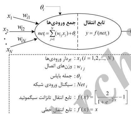
شکل ۱. ساختار یک نرون از شبکه عصبی مصنوعی.
