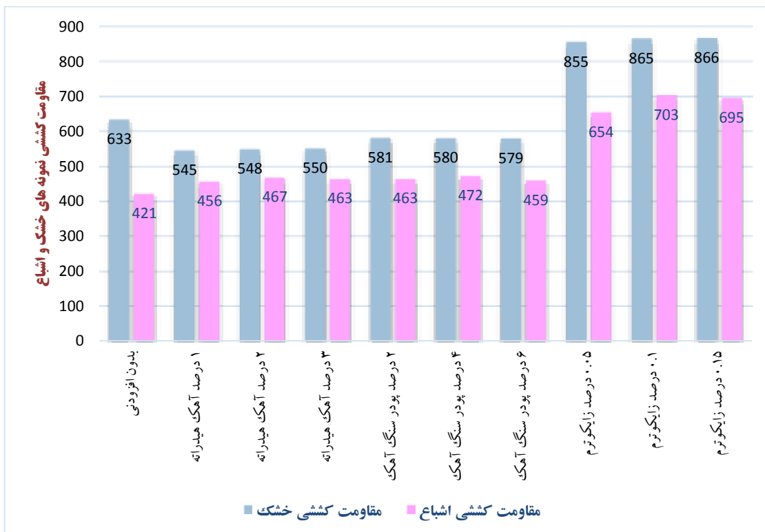
شکل ۶. نتایج مقاومت کشی خشک و اشباع برای مخلوط آسفالتی نوع C
