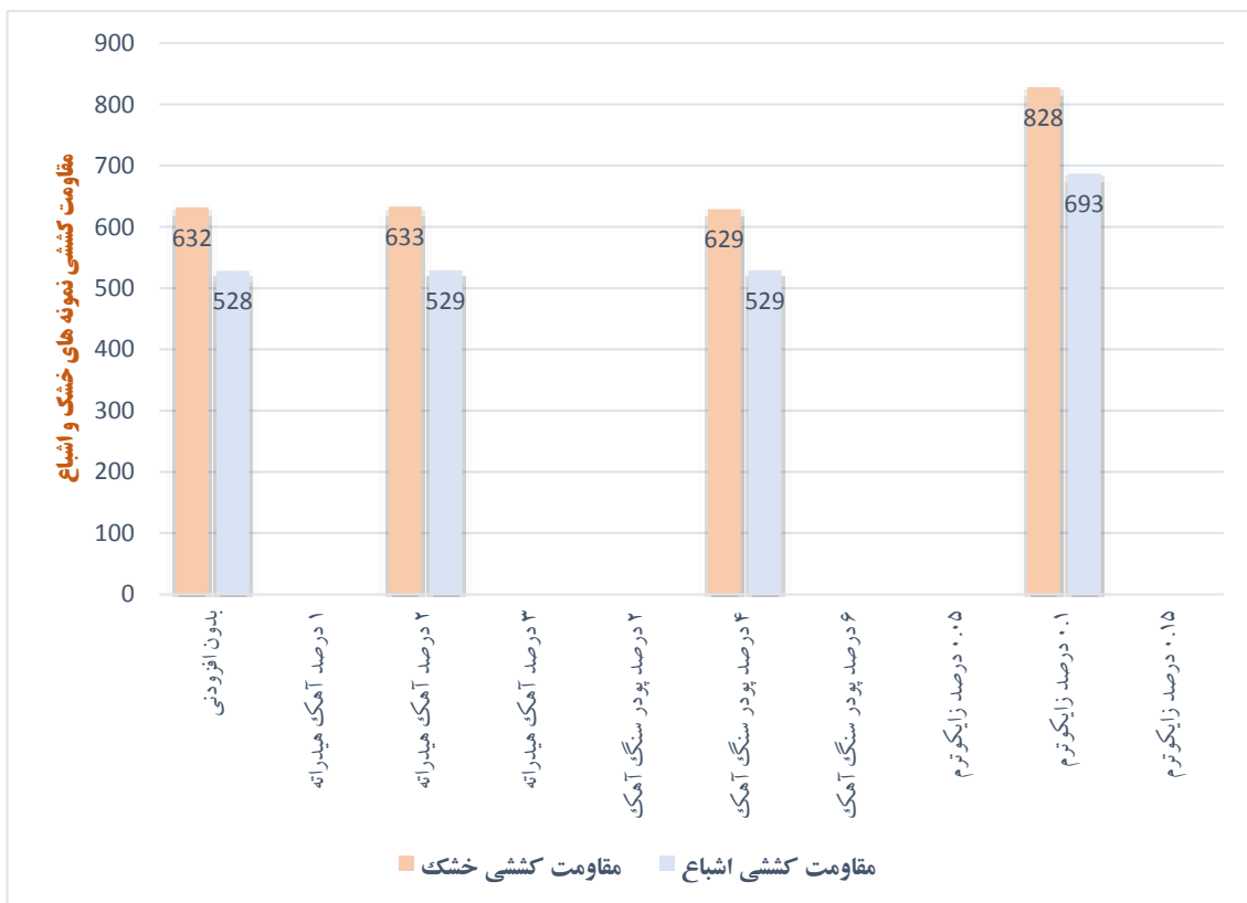
شکل ۵. نتایج مقاومت کشی خشک و اشباع برای مخلوط آسفالتی نوع B
