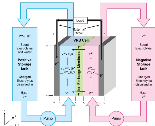
شکل (۱): مکانیزم عملکرد باتری جریان و انادیومی
