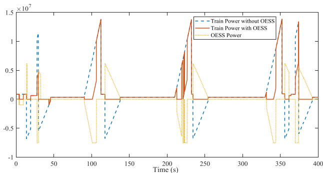
شکل (۷): نمودار توان یک قطار در دو حالت با و بدون سیستم ذخیره‌ساز و توان سیستم ذخیره‌ساز
