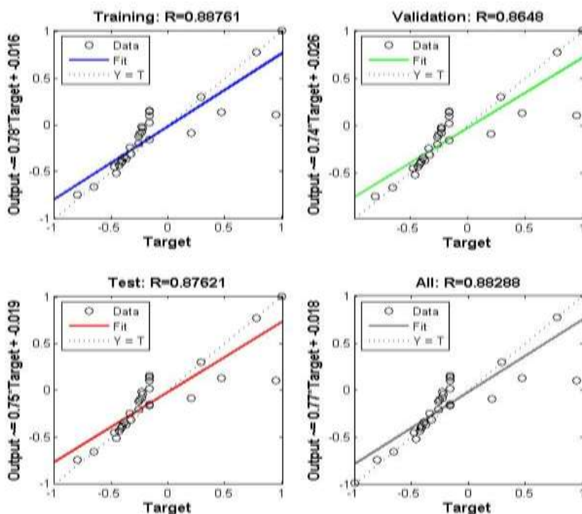
شکل (۳): رگرسیون داده‌ها در شبکه عصبی پرسپترون بوت استرپ شده برای مدل شاخص بارپذیری شبکه در پخش بار بهینه شبکه ۳۰ شین IEEE
