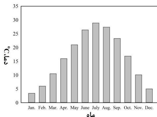
ب. میانگین ماهیانه متوسط دمای برج خشک
