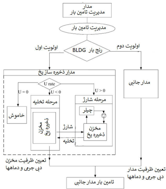
شکل (۴): طرح‌واره عملیاتی و مدل اجرایی سیستم ذخیره‌سازی سرما در یخ در نرم‌افزار انرژی پلاس [۶]
