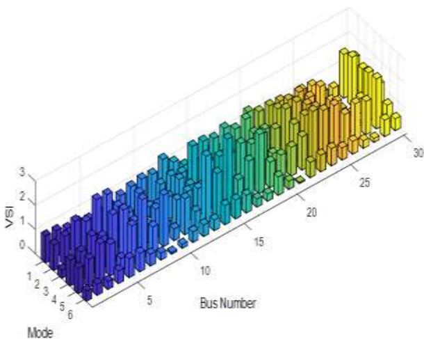
شکل (۱۱): مقایسه شاخص پایداری ولتاژ به‌ازای شش حالت
