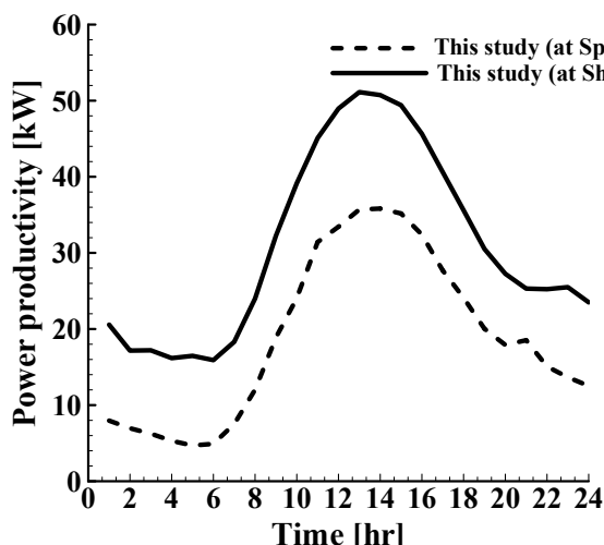
شکل (۵): مقایسه توان تولیدی شهرهای شیراز و مازانارس اسپانیا در طول روز ۲ سپتامبر
