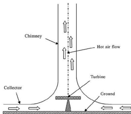
شکل (۱): طرح‌وارهٔ یک نیروگاه دودکش خورشیدی [۱۶]
