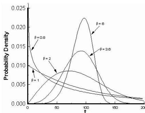
شکل (۵): توزیع دو پارامتری وایبل
