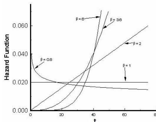
شکل (۶): تغییرات تابع خرابی
