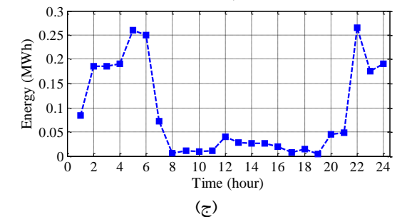
شکل (۴): تأمین انرژی توسط تجمیع‌گر مورد مطالعه، (الف) از بازار روز آینده، (ب) از بازار تعادل مثبت و (ج) از بازار تعادل منفی.
