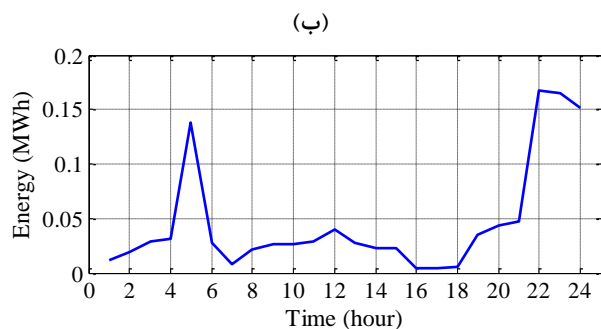
شکل ۸: تأمین انرژی توسط تجمیع گر مورد مطالعه، (الف) از بازار روز آینده، (ب) از بازار تعادل مثبت و (ج) از بازار تعادل منفی
