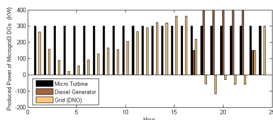
شکل (۱۲): وضعیت تولید واحدهای تولید پراکنده در ریزشکه سوم قبل از باز تنظیم توان در طرح اول
