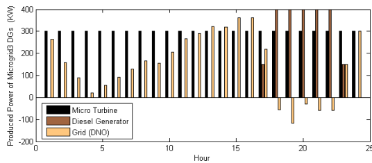
شکل (۱۷): وضعیت تولید واحدهای تولید پراکنده در ریزشبكة سوم بعد از باز تنظیم توان در طرح اول
