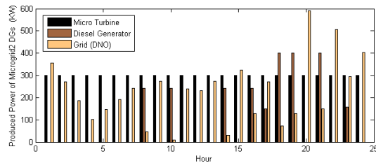
شکل (۲۵): وضعیت تولید واحدهای تولید پراکنده در ریزشبکه دوم بعد از باز تنظیم توان در طرح دوم
