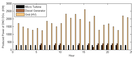
شکل (۱۸): وضعیت تولید واحدهای تولید پراکنده در شبکه توزیع بعد از باز تنظیم توان در طرح اول
