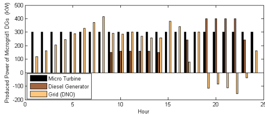
شکل (۲۴): وضعیت تولید واحدهای تولید پراکنده در ریزشبکه اول بعد از باز تنظیم توان در طرح دوم
