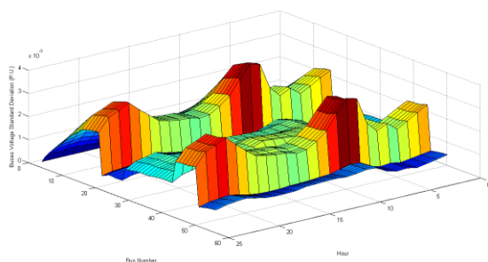
شکل (۲۵): وضعیت انحراف معیار ولتاژ ۵۳ باس شبکه قبل از باز تنظیم توان در طرح دوم
