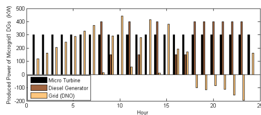
شکل (۱۰): وضعیت تولید واحدهای تولید پراکنده در ریزشکه اول قبل از باز تنظیم توان در طرح اول
