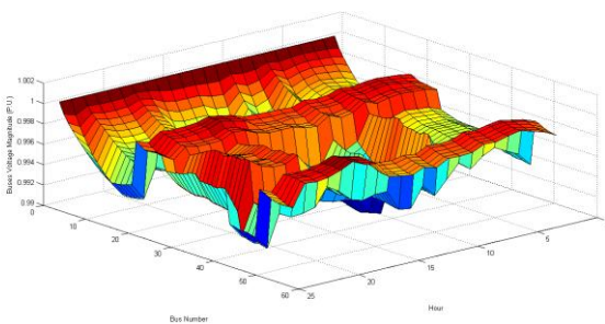
شکل (۱۹): وضعیت دامنه ولتاژ ۵۳ باس شبکه بعد از باز تنظیم توان در طرح اول
