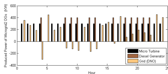
شکل (۱۱): وضعیت تولید واحدهای تولید پراکنده در ریزشکه دوم قبل از باز تنظیم توان در طرح اول
