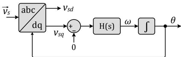
شکل (۳): بلوک دیاگرام SRF-PLL
