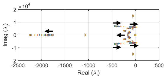
الف) مقادير ویژه سيستم
