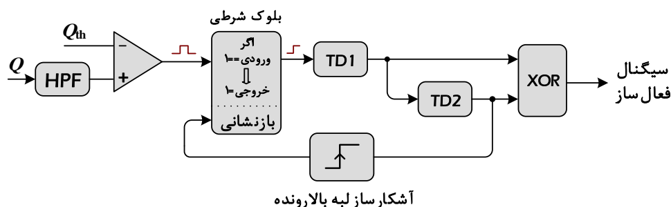
شکل (۵): ساختار واحد تولیدکننده‌ی سیگنال فرمان آغاز فرآیند اصلاح مشخصه افقی
