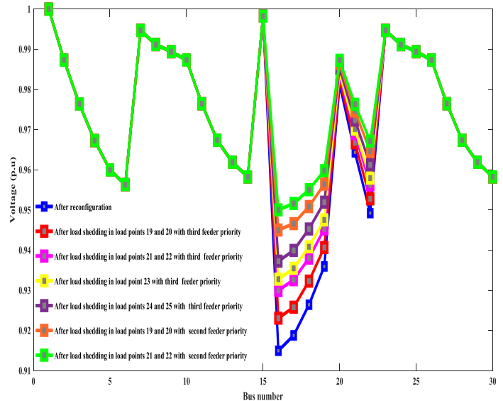
شکل (۸) - پروفیل ولتاژ قبل و بعد از دوره بازیابی بار برای سناریو سوم - مورد ۲
