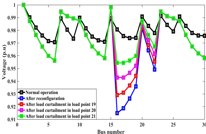
شکل (۳) - پروفیل ولتاژ قبل و بعد از دوره بازیابی بار برای سناریو اول - مورد ۱
