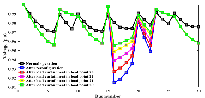
شکل (۴) - پروفیل ولتاژ قبل و بعد از دوره بازیابی بار برای سناریو اول - مورد ۲
