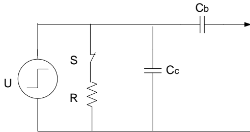
شکل ۲. مدار مولد پالس تخلیه جزئی
