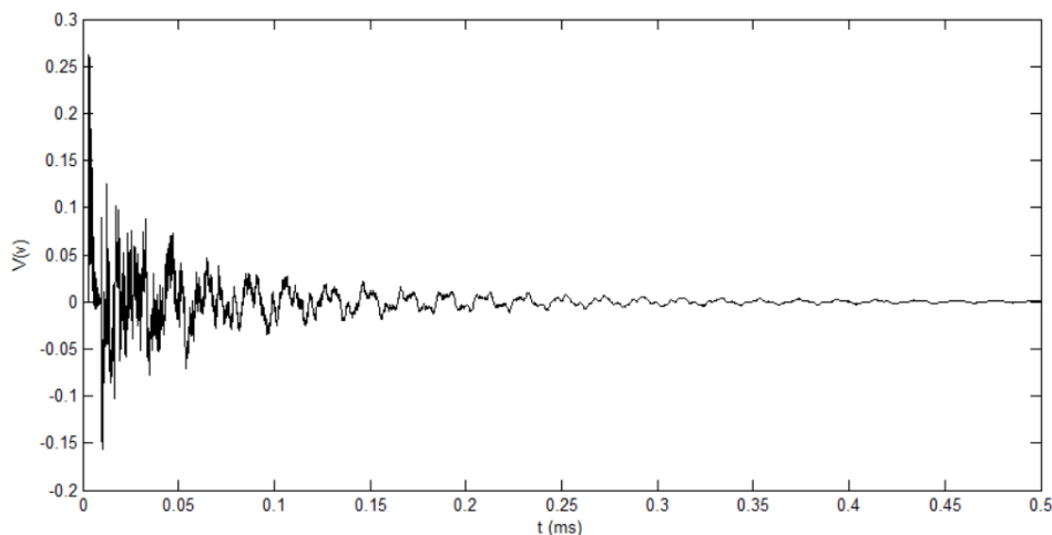
شکل ۷. سیگنال ضبط شده در انتهای خط ناشی از اعمال پالس در محل تیر اول
