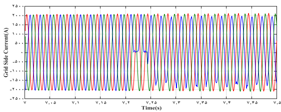
شکل (۱۷): جریان سه فاز مبدل سمت شبکه با رخداد خطا در سوئیچ پایین فاز B با کنترل تحمل‌پذیر خطای پیشنهادی
