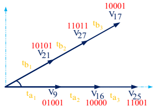
شکل (۶): برداری تشکیل دهنده ی سکتور اول
