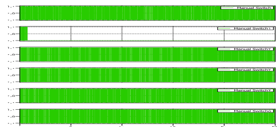
شکل (۱۲): نمونه‌ی سیگنال ورودی به گیت IGBTها در مبدل سمت
