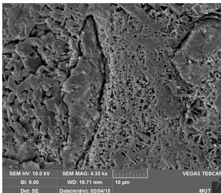
شکل ۷- ریزساختار زمینه حاوی ۰.۵٪ افزودنی بورات آلومینیوم پس از پخت در ۱۵۵۰ °C
