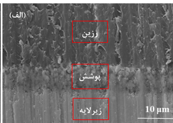
شکل ۴- تصاویر میکروسکوپ الکترونی از مقاطع عرضی نمونه‌های پوشش داده شده در حمام‌های الف) نمونه ۱، ب) نمونه ۲.
