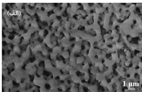
شکل ۳- تصاویر میکروسکوپ الکترونی نمونه‌های پوشش داده شده در حمام‌های الف) نمونه ۱، ب) نمونه ۲.
