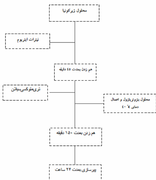
شکل ۱- شماتیک مراحل تهیه محلول هیبریدی
