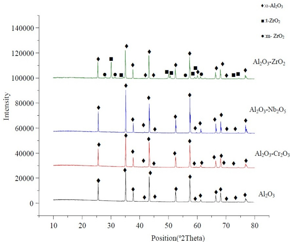
شکل ۲- الگوهای پراش نمونه‌های تف جوشی شده در دمای 1500^\circ\text{C}
