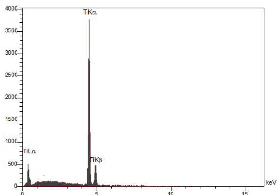
شکل ۹- آنالیز طیف‌سنجی پراش انرژی پرتو ایکس نقطه B مشخص شده در شکل (۷، ج).
