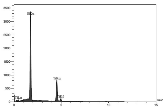
شکل ۱۰- آنالیز طیف‌سنجی پراش انرژی پرتو ایکس نقطه C مشخص شده در شکل (۷، ج).
