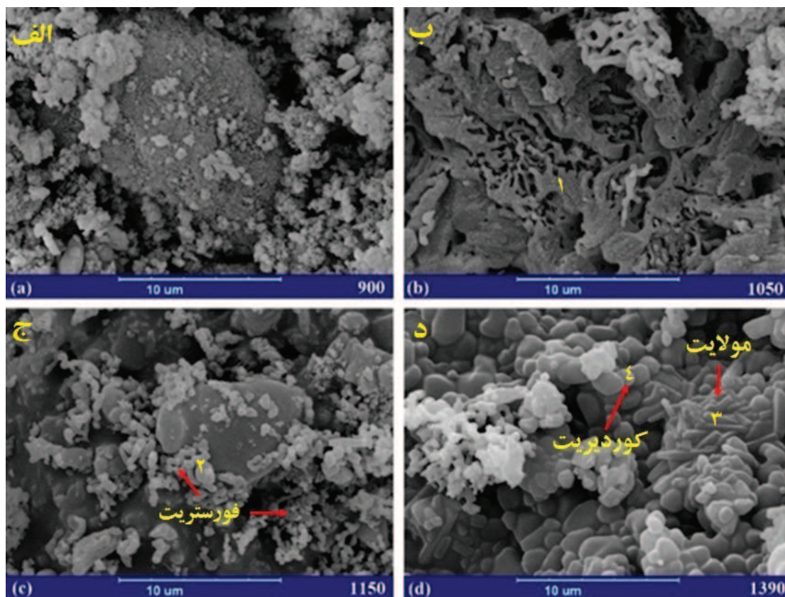
شکل ۴- تصاویر میکروسکوپ الکترونی روبشی از مخلوط پودری شامل (۳۲/۹۸ درصد وزنی) nano-SiO_2 ، (۲۲/۳۸ درصد وزنی) Al_2O_3 و (۴۴/۶۴ درصد وزنی) MgCl_2 \cdot 6H_2O که در دماهای (الف) ۹۰۰، (ب) ۱۰۵۰، (ج) ۱۱۵۰ و (د) 1390^{\circ}C به مدت ۳ ساعت حرارت دهی شده است.
