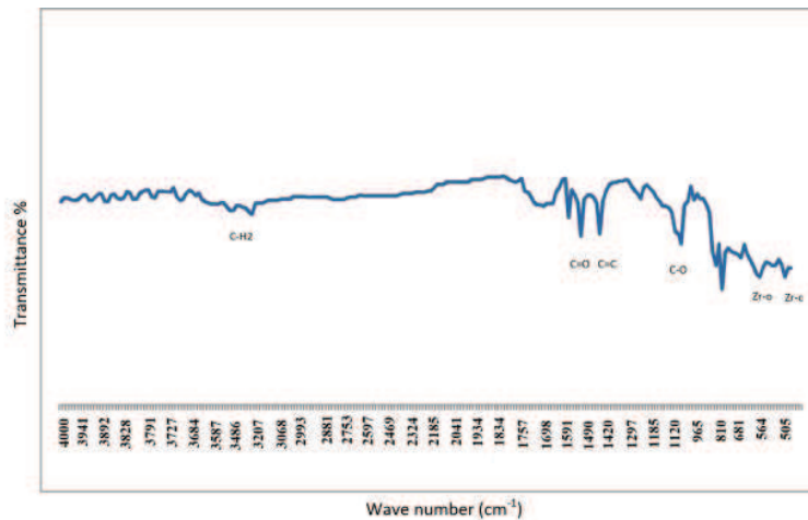
شکل ۵- طیف FTIR از نمونه پودری حاصل از فرایند عملیات حرارتی در دمای ۷۰۰ °C و pH=۵
