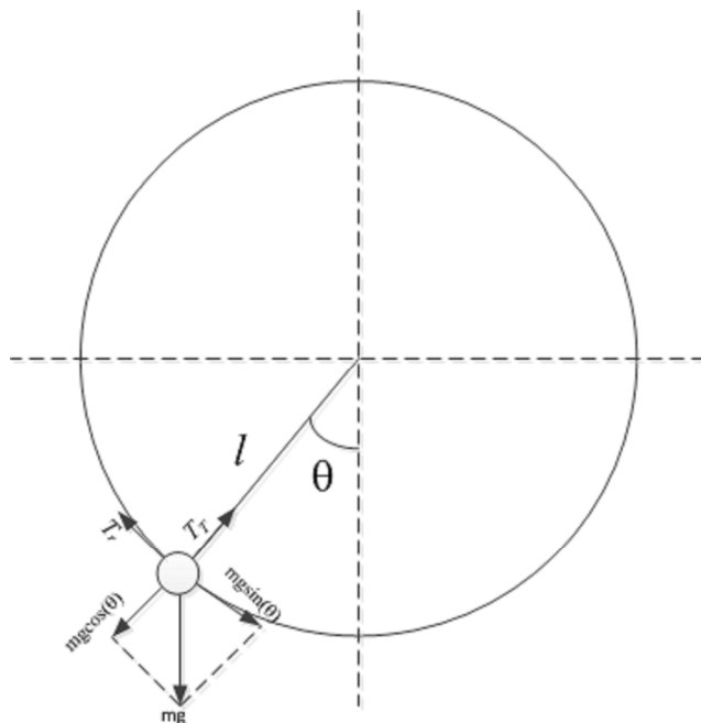
شکل ۴: دیاگرام آزاد آونگ متصل به شفت.
