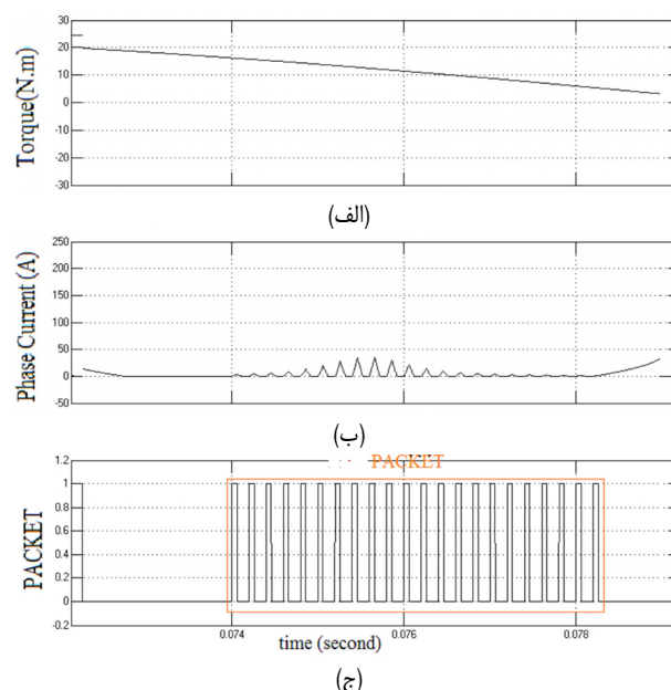
شکل ۸: بزرگ‌نمایی منحنی‌ها در ناحیه ۲، (الف) منحنی گشتاور بار، (ب) منحنی جریان فاز و (ج) خروجی برد تشخیص.
