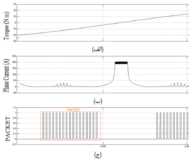
شکل ۷: بزرگ‌نمایی منحنی‌ها در ناحیه ۱، (الف) منحنی گشتاور بار، (ب) منحنی جریان فاز و (ج) خروجی برد تشخیص.
